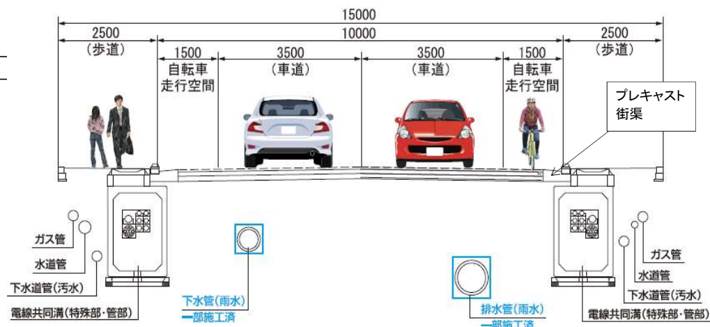
標準横断面
